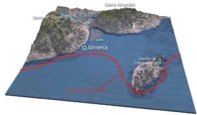
2 HACE 1,8 MILLONES DE AÑOS
