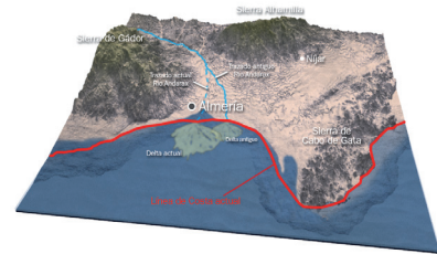
3 HACE 0,9 MILLONES DE AÑOS
