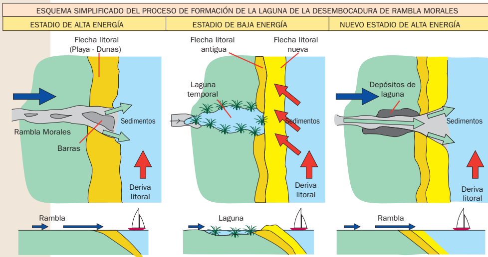
Laguna que se forma detrás de la flecha litoral.
