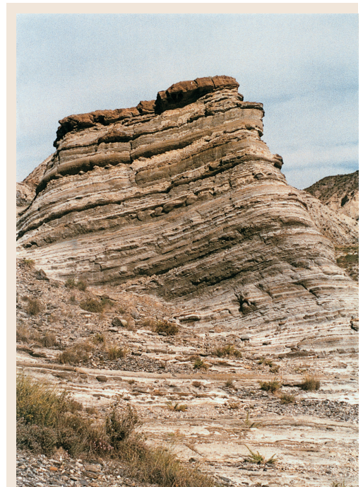
Secuencia turbidítica del Desierto de Tabernas.
