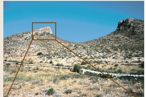
Estructura de los antiguos canales que conectaban con el espolón
