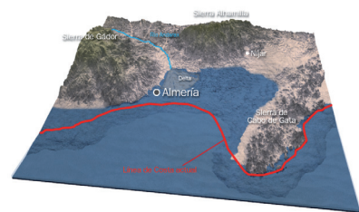
3 HACE 0,9 MILLONES DE AÑOS
